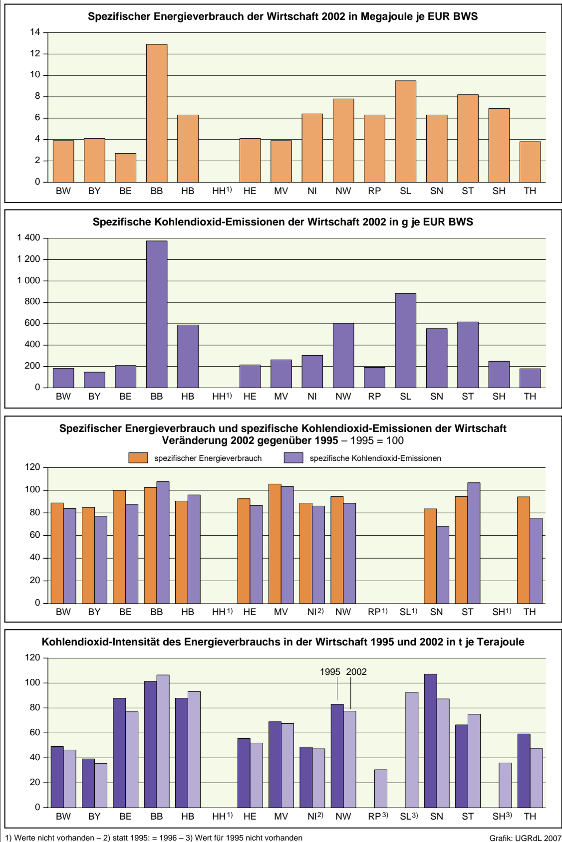
Abb. 13 Energieverbrauch und Kohlendioxid-Emissionen der Wirtschaft
